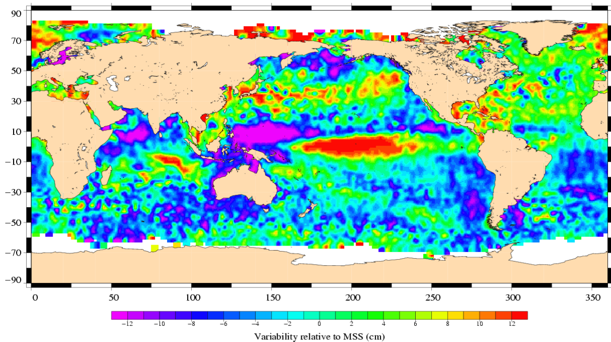
Envisat Cycle 010 30/09/2002 – 04/11/2002
