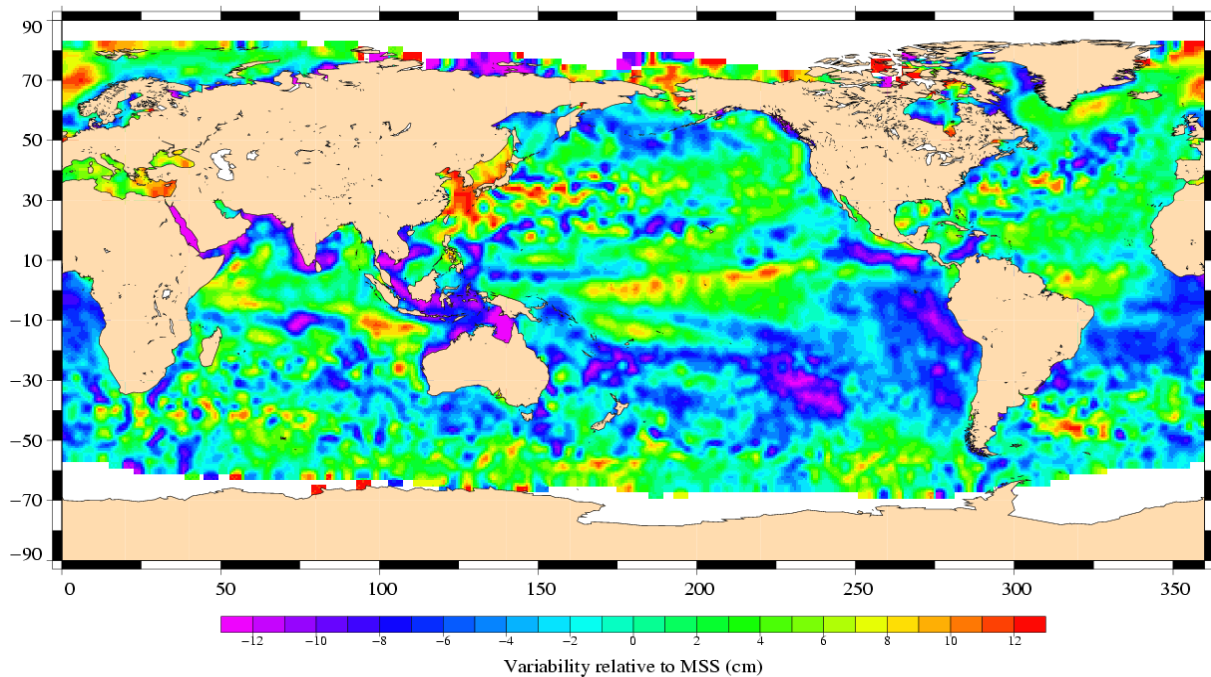
Envisat Cycle 029 26/07/2004 – 30/08/2004
