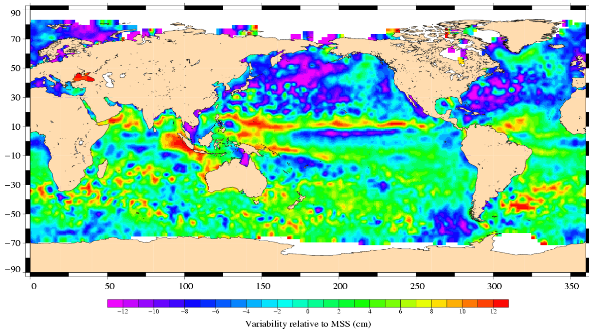
Envisat Cycle 037 02/05/2005 – 06/06/2005
