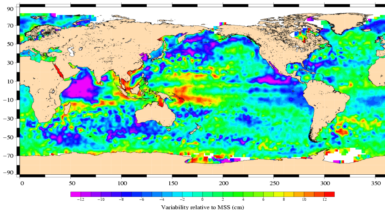
Envisat Cycle 043 28/11/2005 – 02/01/2006
