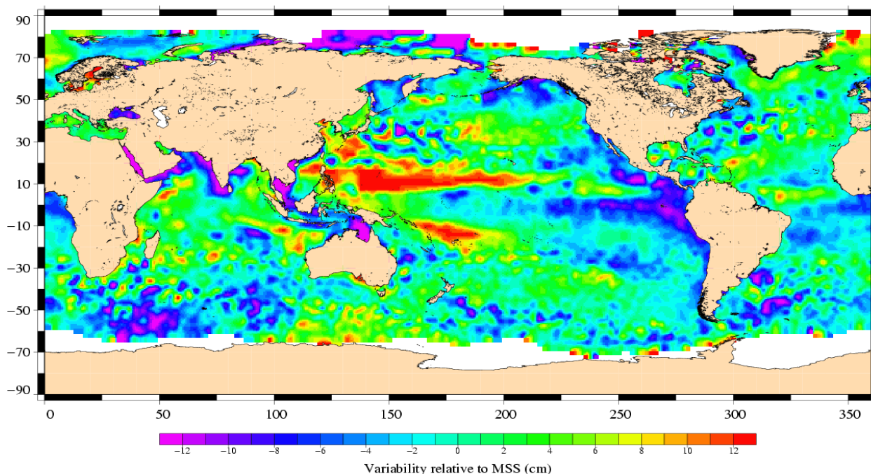
Envisat Cycle 060 16/07/2007 – 20/08/2007
