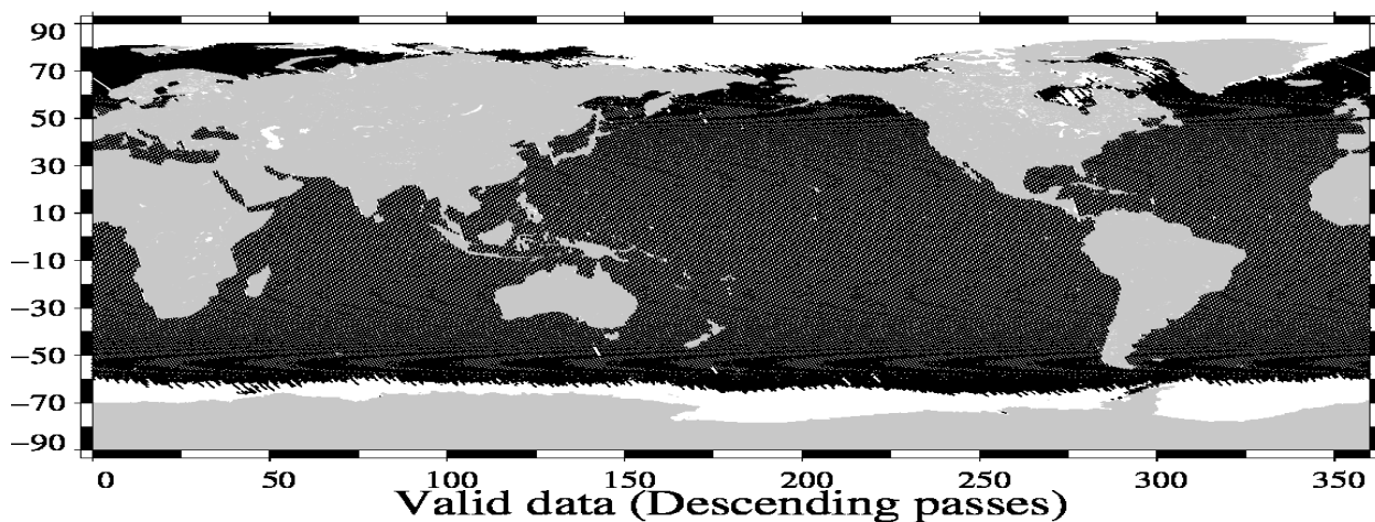
Valid data (Descending passes) Envisat Cycle 104 (24/06/2011 / 24/07/2011)
