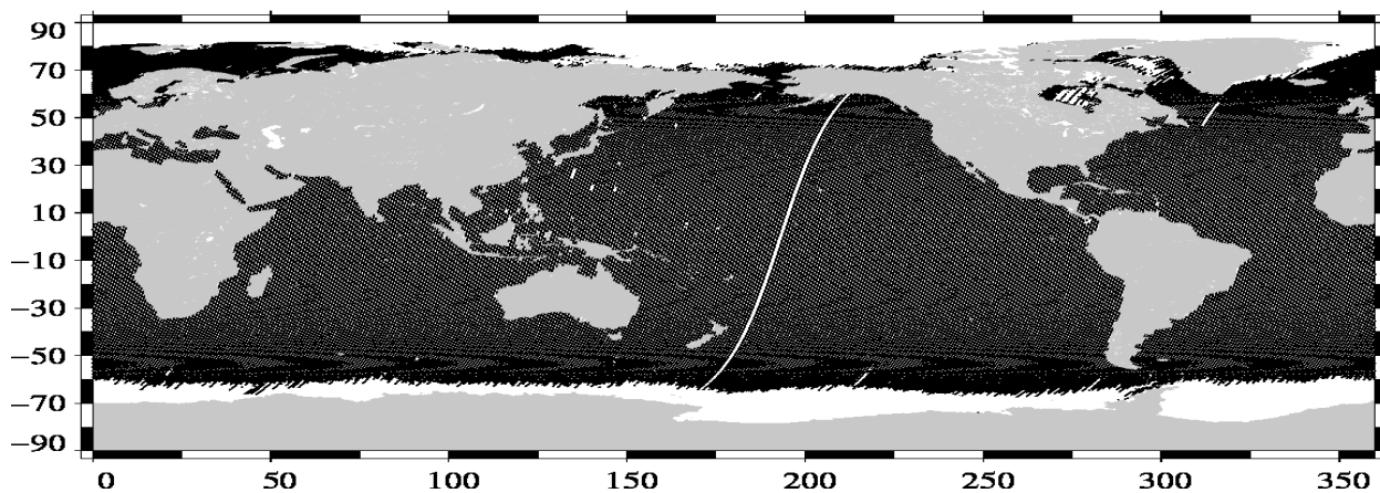
Valid data (Descending passes) Envisat Cycle 104 (24/06/2011 / 24/07/2011)
