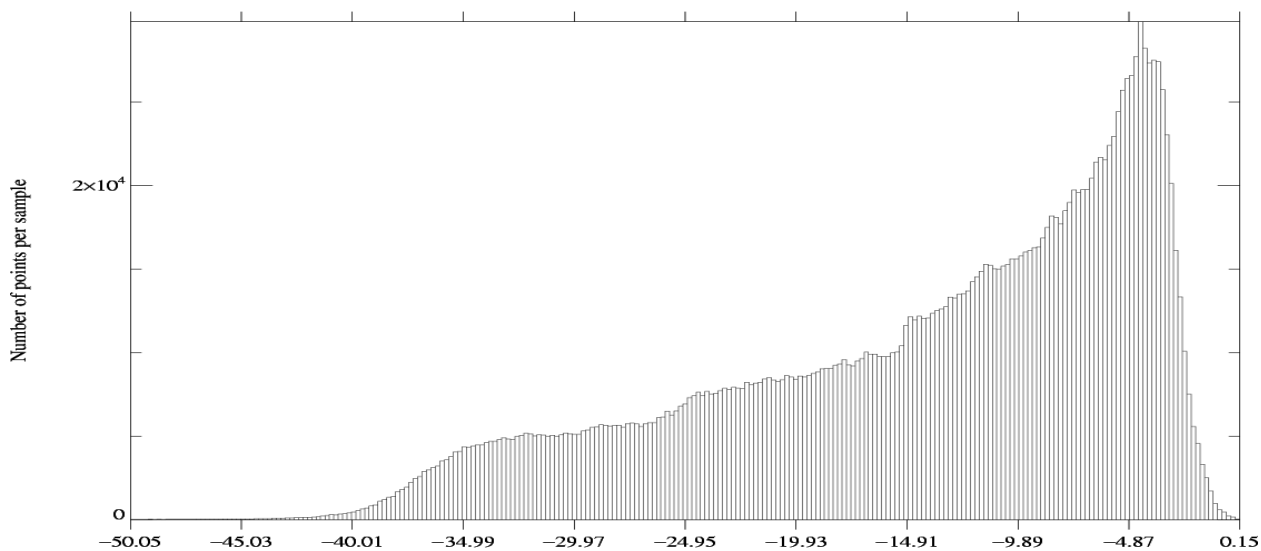
Jason-1 Radiometer wet tropospheric correction ( unit : cm)
