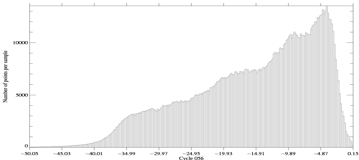
Envisat Radiometer wet tropospheric correction, |Latitude|<66 ( unit : cm)
