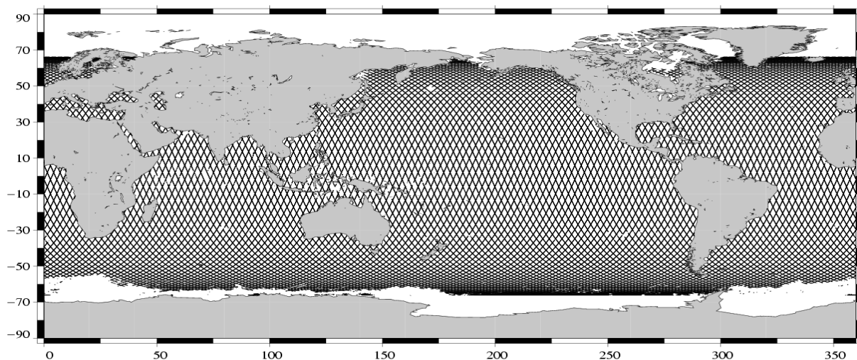
Valid data Jason-1 Cycle 070 (30/11/2003 / 10/12/2003)
