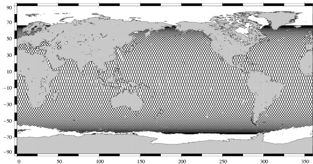
Valid data Jason-1 Cycle 107 (01/12/2004 / 11/12/2004)
