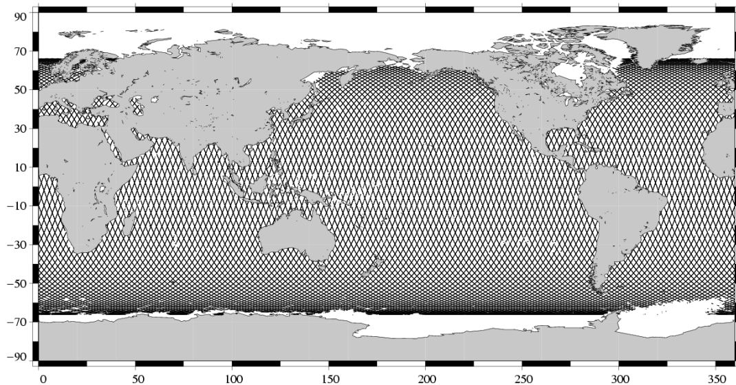
Valid data Jason-1 Cycle 109 (21/12/2004 / 31/12/2004)
