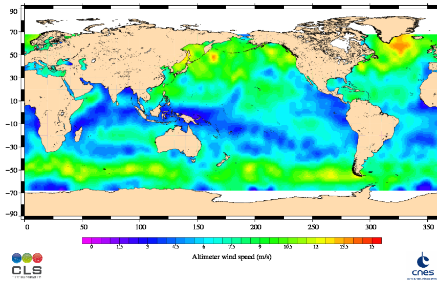
Jason-1 Cycle 256 17/12/2008 - 27/12/2008
