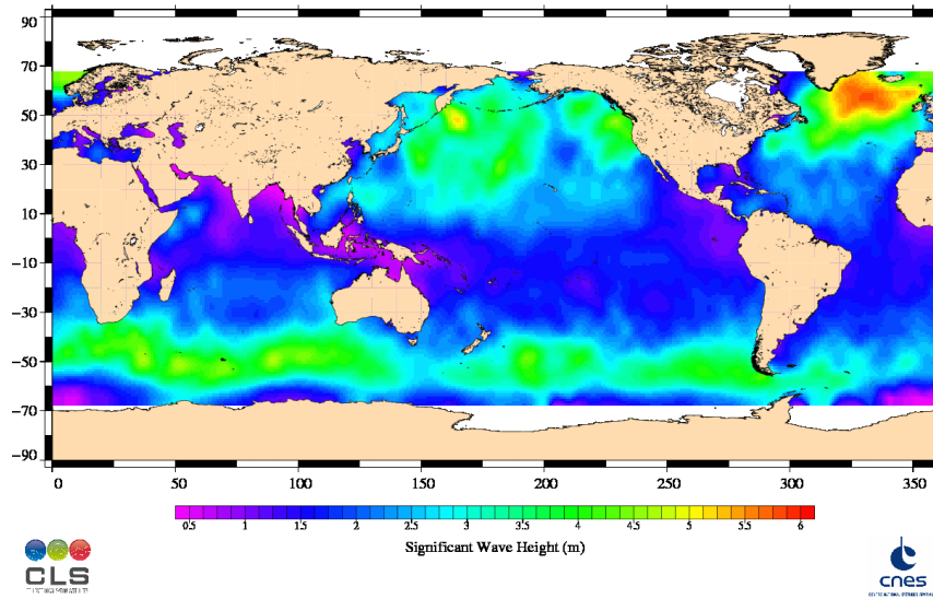
Jason-1 Cycle 256 17/12/2008 - 27/12/2008
