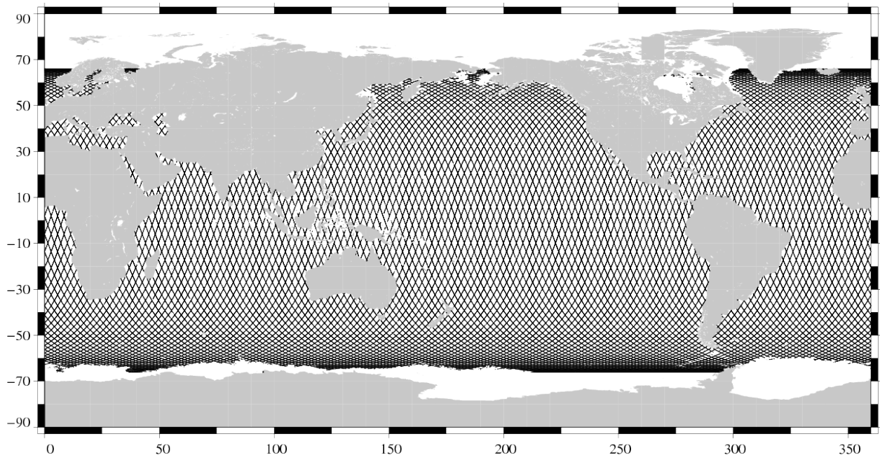
Valid data Jason-1 Cycle 309 (22/05/2010 / 01/06/2010)
