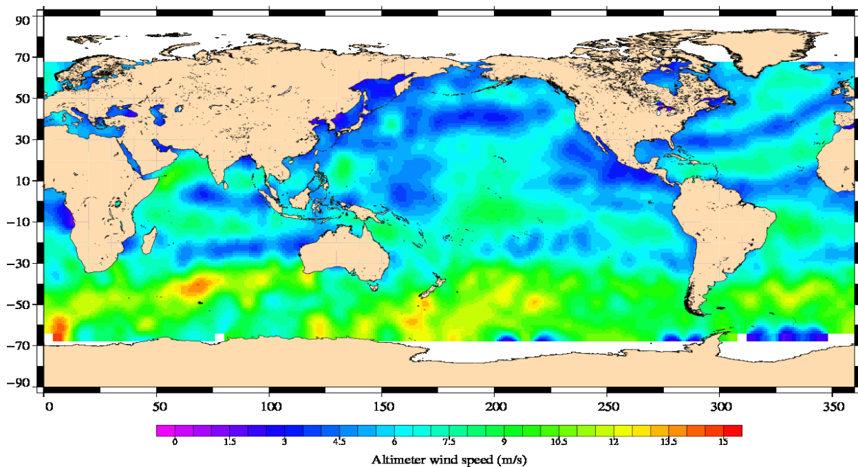
Jason-1 Cycle 352 22/07/2011 - 01/08/2011
