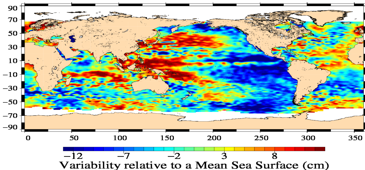
Jason-1 Cycle 362 29/10/2011 – 08/11/2011
