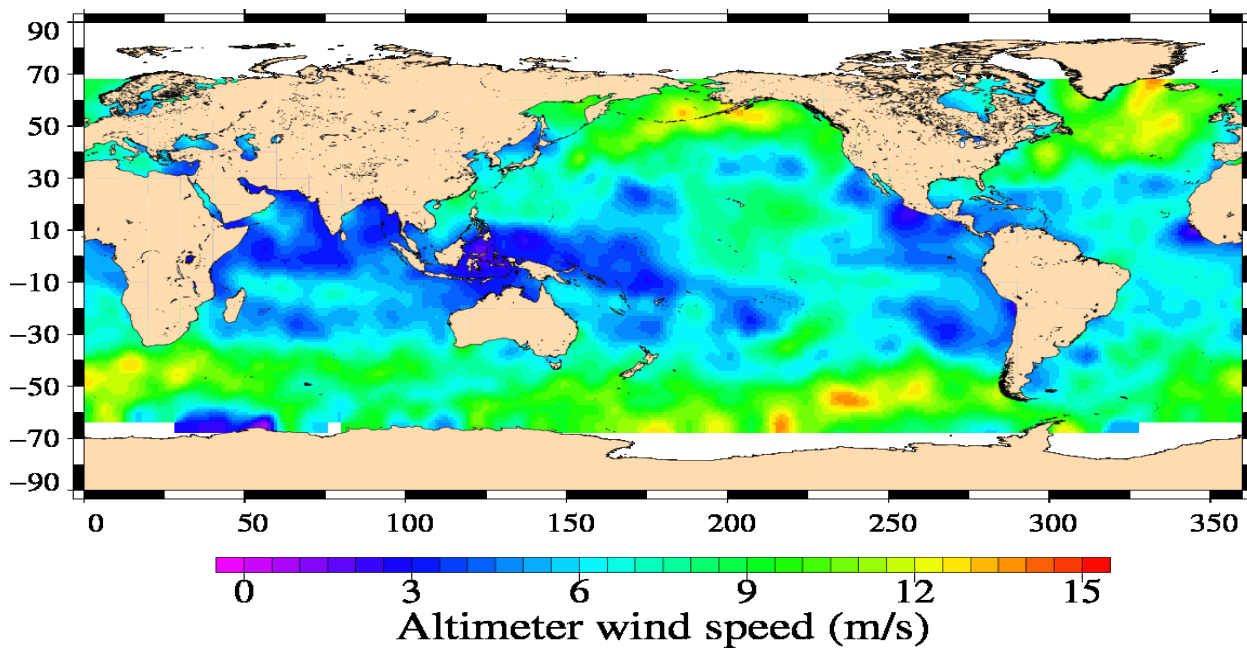
Jason-1 Cycle 362 29/10/2011 – 08/11/2011
