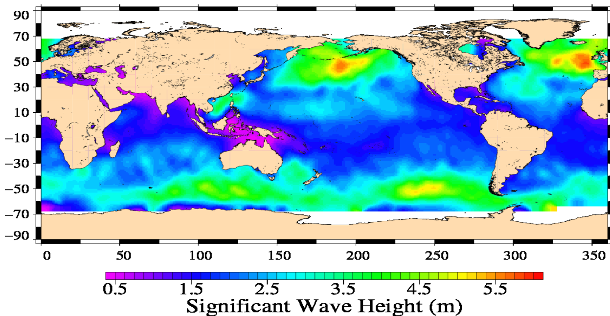
Jason-1 Cycle 366 08/12/2011 – 18/12/2011
