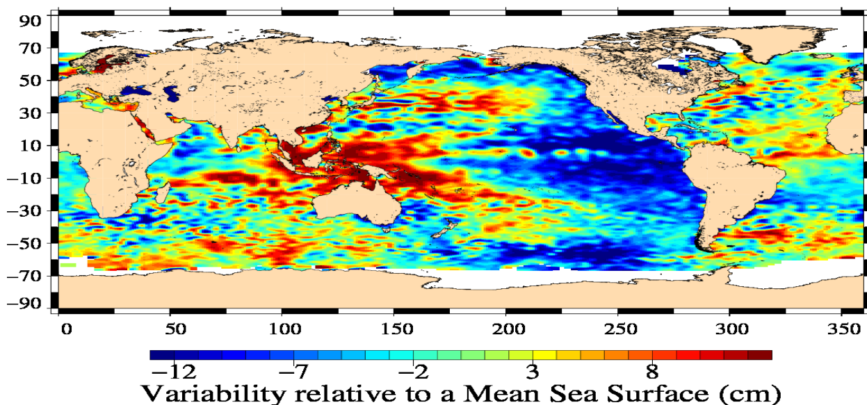
Jason-1 Cycle 366 08/12/2011 – 18/12/2011
