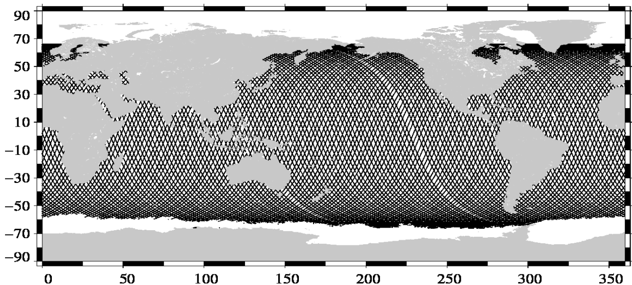
Valid data Jason-1 Cycle 516 (29/10/2012 / 08/11/2012)
