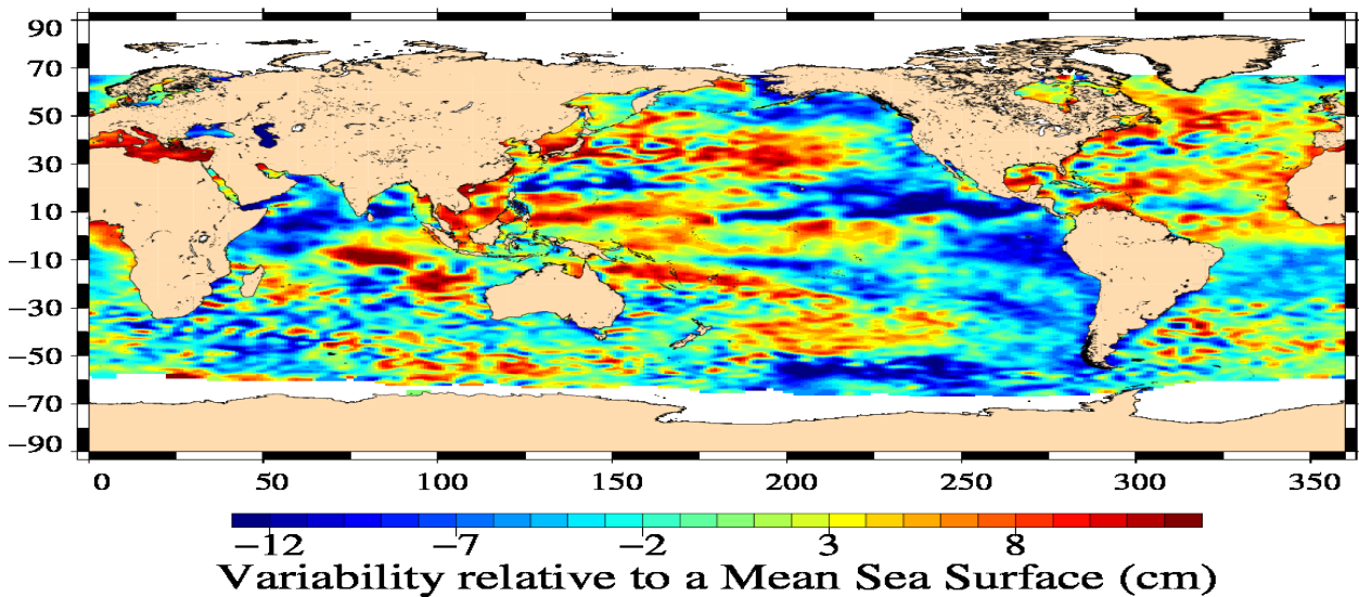
Jason-1 Cycle 516 29/10/2012 – 08/11/2012
