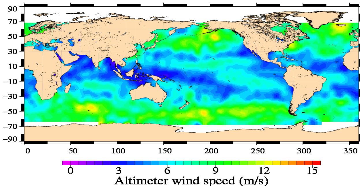
Jason-1 Cycle 516 29/10/2012 – 08/11/2012
