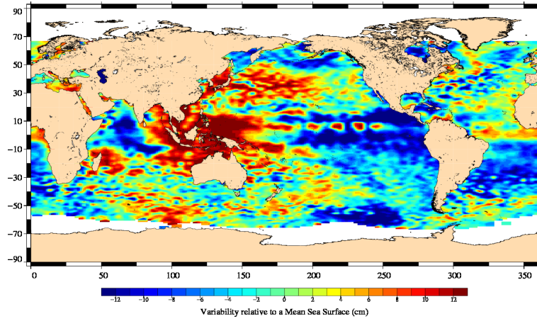
Jason-2 Cycle 086 01/11/2010 - 11/11/2010
