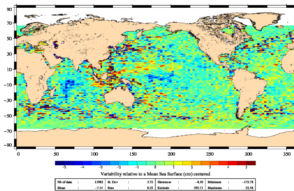
Jason-1 – Jason-2 (Cycle 022 to 089)
