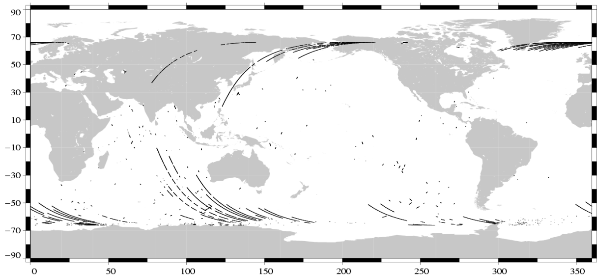
Edited parameter : Radiometer wet tropospheric correction T/P Cycle 395 (04/06/2003 / 14/06/2003)
