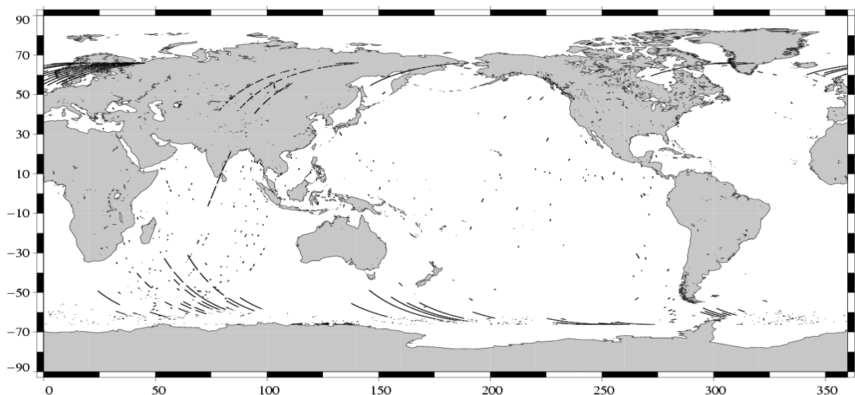
Edited parameter : Radiometer wet tropospheric correction T/P Cycle 401 (03/08/2003 / 13/08/2003)
