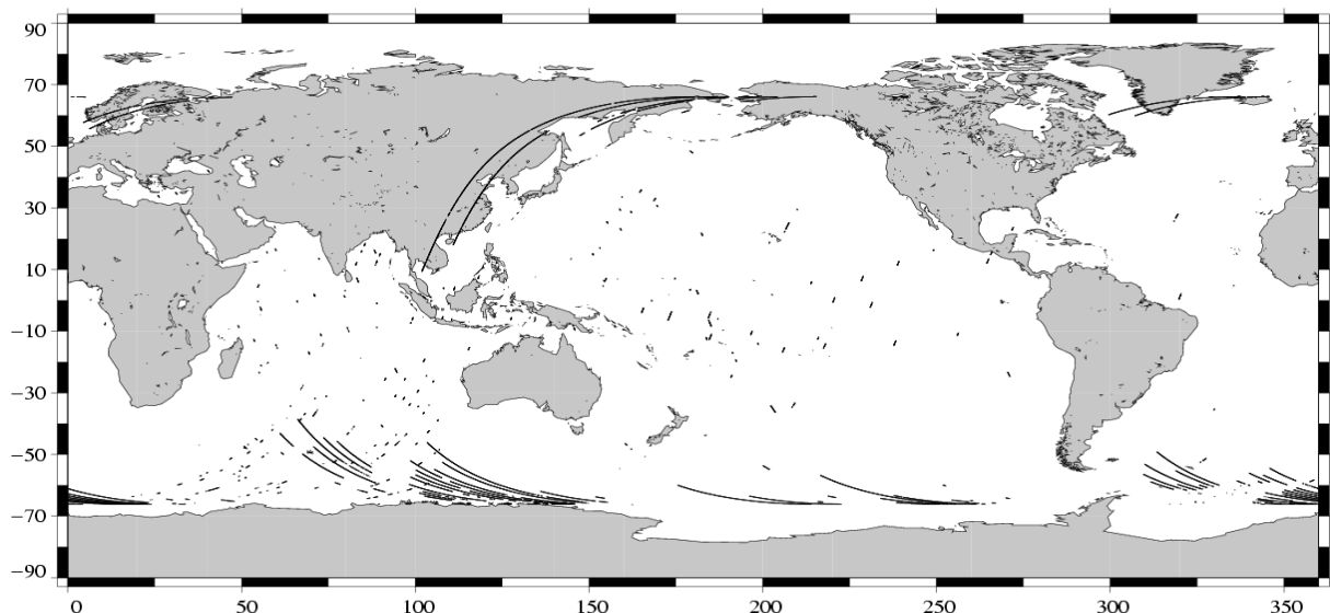
Edited parameter : Radiometer wet tropospheric correction T/P Cycle 416 (30/12/2003 / 09/01/2004)
