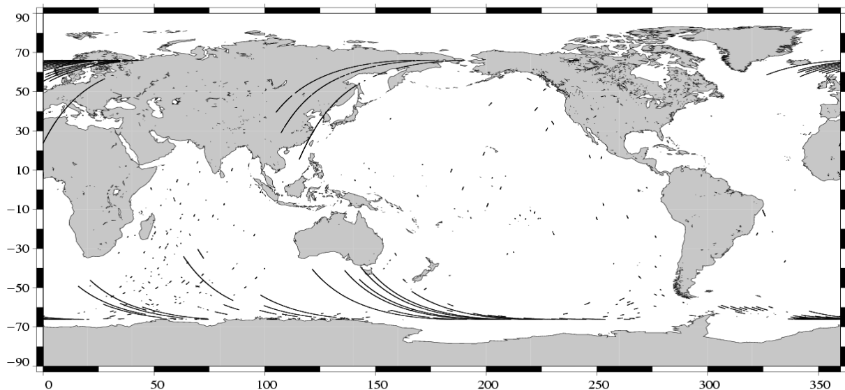
Edited parameter : Radiometer wet tropospheric correction T/P Cycle 417 (09/01/2004 / 18/01/2004)
